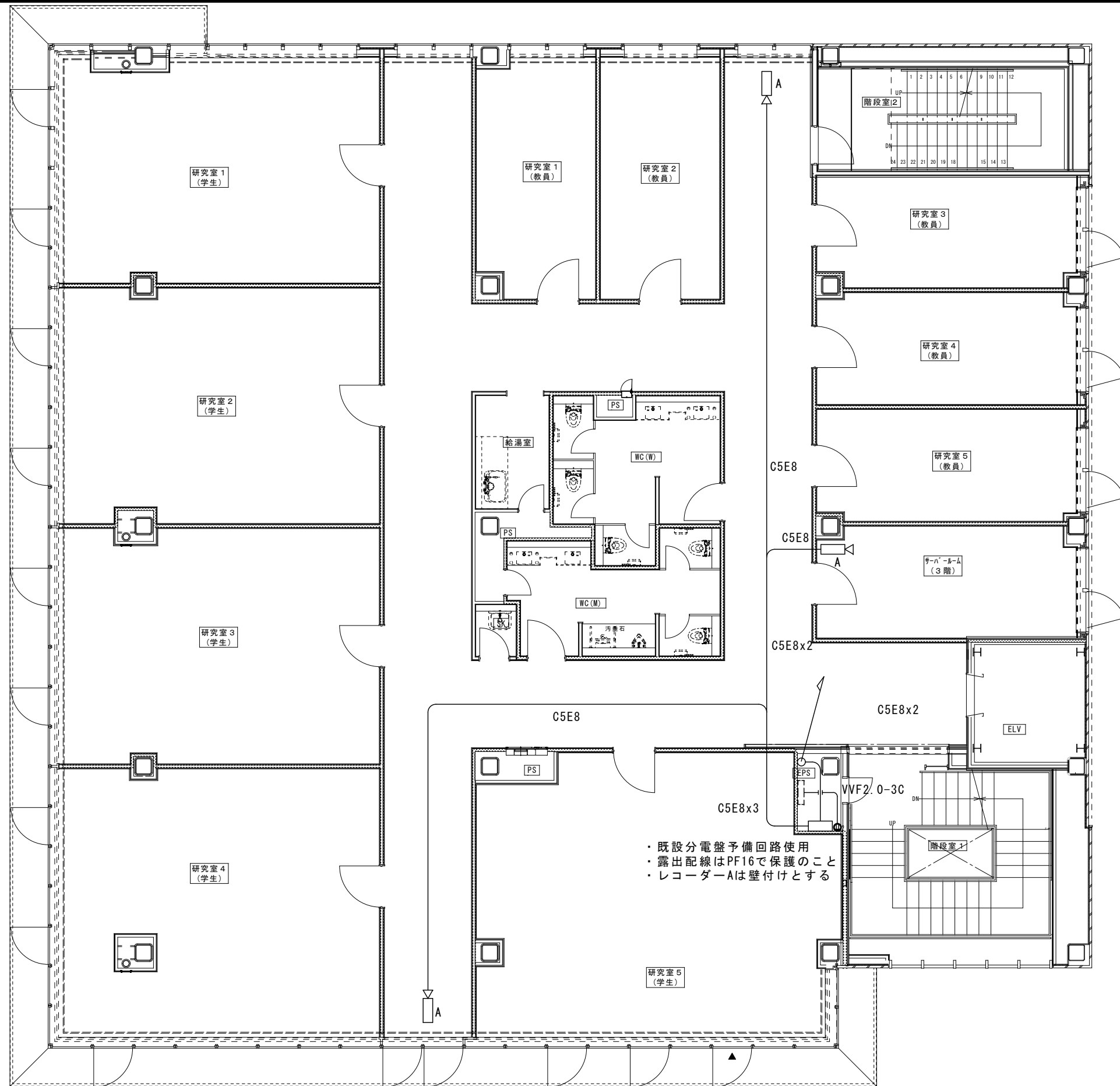
3階平面図
